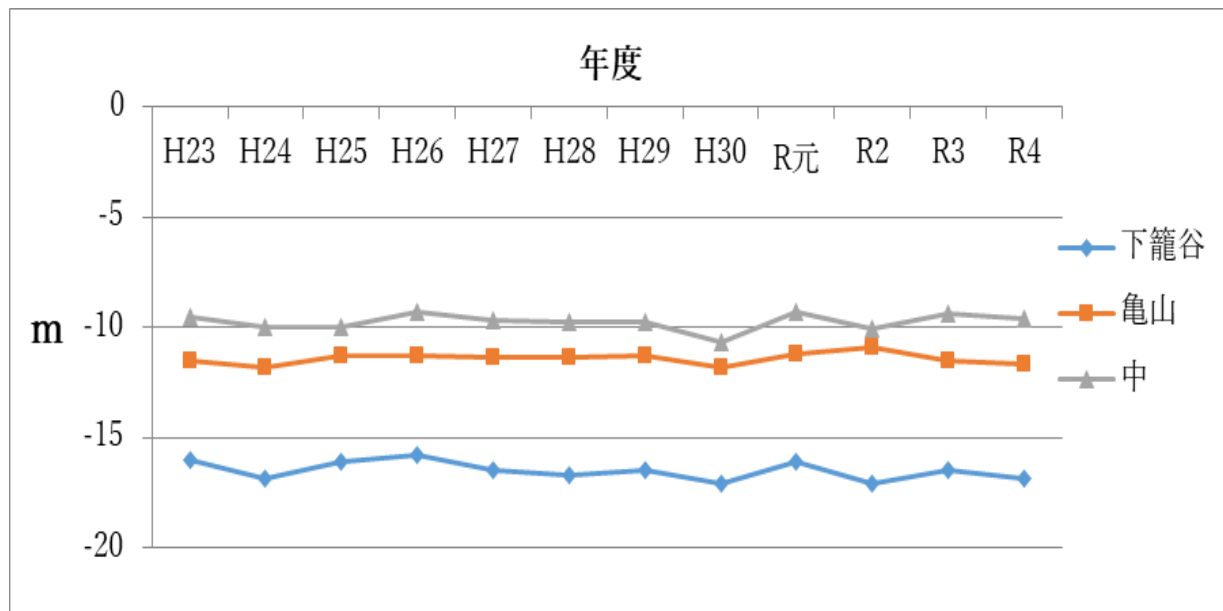
図 3. 浅井戸地下水位の経年変化（3 月）
