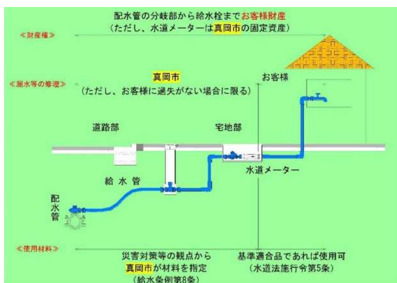
図 5.5 給水装置の維持管理区分
