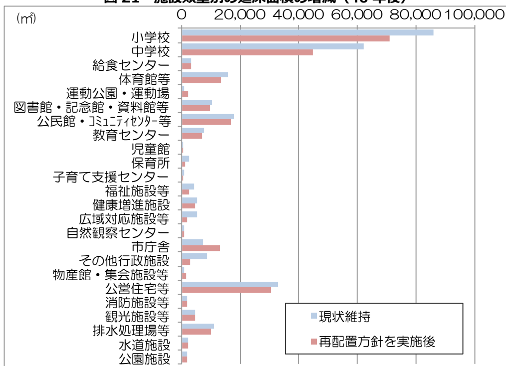
図 21 施設類型別の延床面積の増減（40年後）
