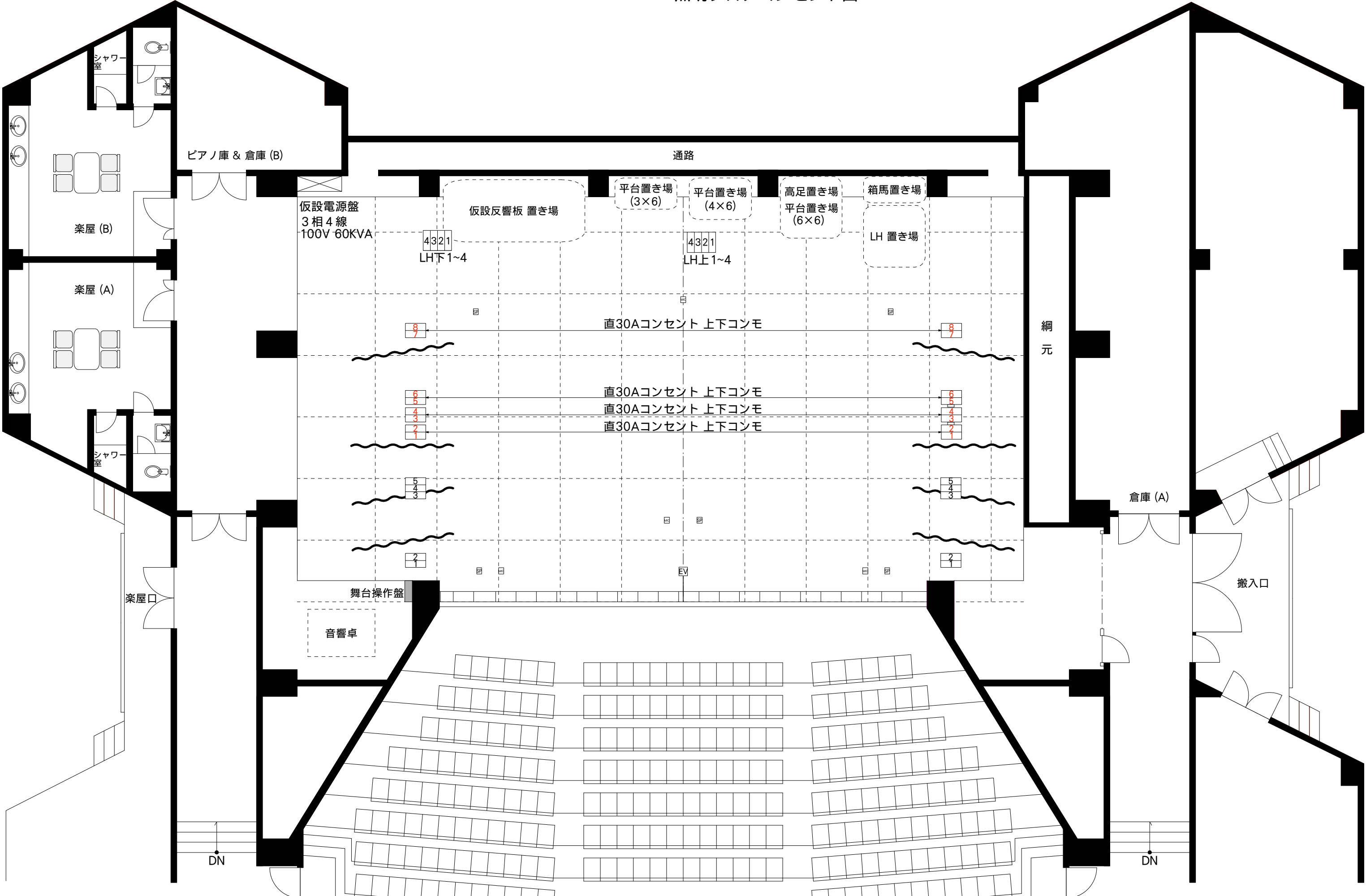
照明フロアコンセント図
