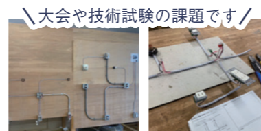
▲第二種電気工事士の技能試験の候補問題 ▲ものづくりコンテスト電気工事部門の作品
